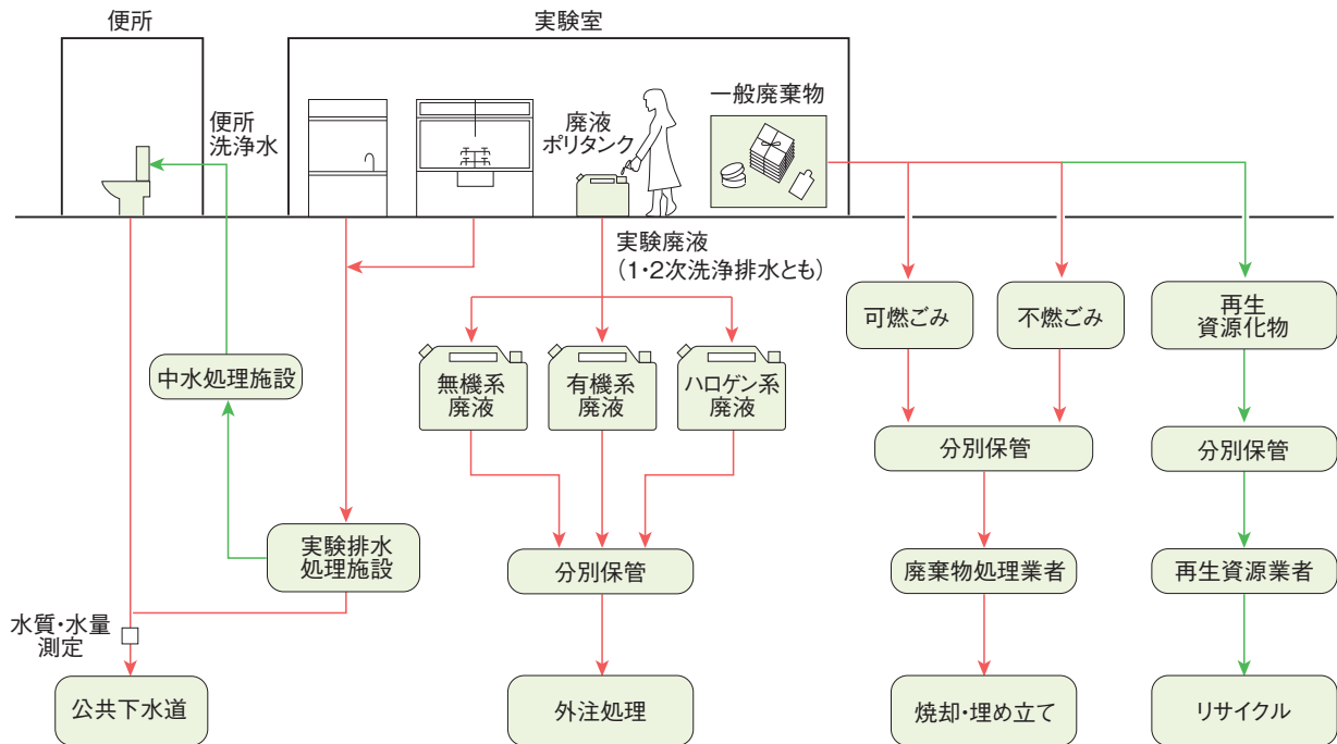
廃棄物・実験排水処理の流れ(岡崎3機関)
