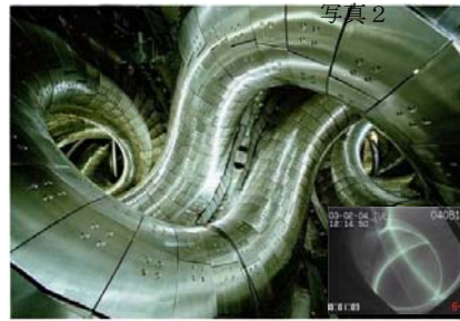
プラズマを閉じ込める磁場のかごを作るLHD内部と閉じ込められたプラズマ(右下。高温のプラズマは目に見える光を出さないで透けて見えます。)
