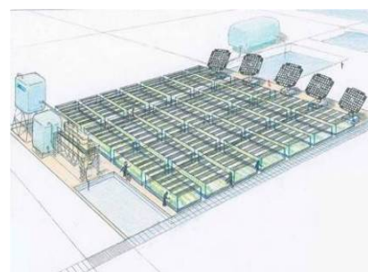
クラスター型太陽集光装置の概要図
