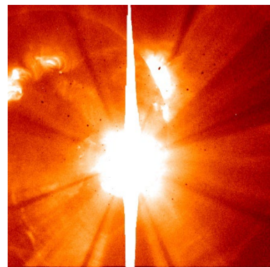
2024年5月11日（日本時間）に発生した X5.8 クラスの大規模フレア（国立天文台/JAXA/MSU）
