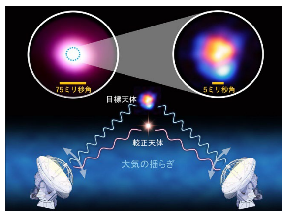
新しい校正手法である「バンド・トゥ・バンド観測誤差補正法」及びうさぎ座R星の概要図
