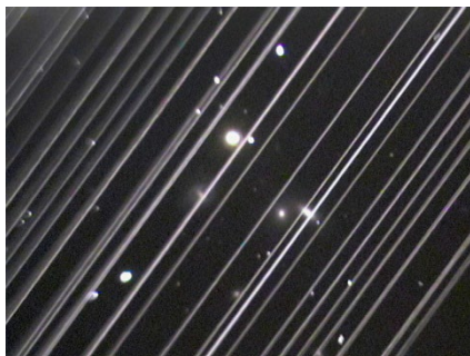
NGC 5353/4 に出現した超新星を撮影中に偶然撮影された Starlink 衛星列による“妨害”。 60 基の衛星群を打ち上げただけでこのような妨害が生じる例 である。
