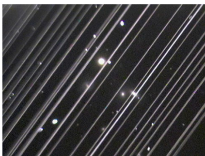
NGC 5353/4 に出現した超新星を撮影中に偶然撮影された Starlink 衛星列による“妨害”。
