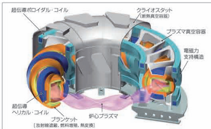
LHD型核融合エネルギー炉FFHR-2m
