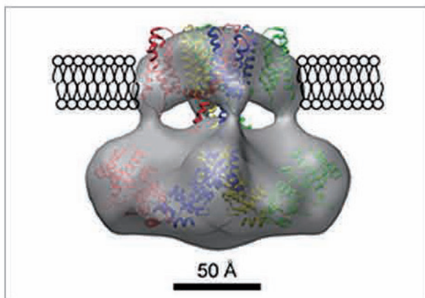
電子顕微鏡で観察したTRPV4チャンネルタンパク質の立体構築モデル
