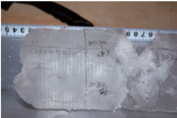
1 [採取された氷床コア] ドームふじ基地で3034.5mの深さの氷床コア（72年前の水）を採取し、過去の地球の環境変動を明らかにする研究が続けられています。
