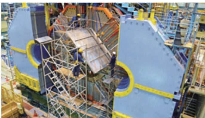
【KEKBによるBelle実験】B中間子の崩壊におけるCP対称性の破れの発見と小林・益川理論の検証など、多くの成果をあげてきました。現在、KEKB加速器及びBelle測定器のアップグレードを進めており、さらなる新しい物理の発見と解明を目指しています。
