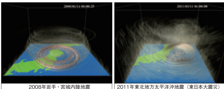
3 データ同化によって再現された大地震に伴う大気変動の様子
