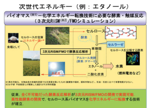
理論・計算科学でセルロース⇒エタノール変換酵素を設計
