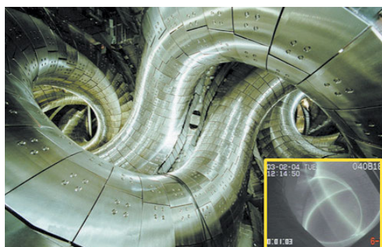
プラズマを閉じ込める磁場のかごを作るLHD内部と閉じ込められたプラズマ(右下。高温のプラズマは目に見える光を出さないので透けて見えます。)
