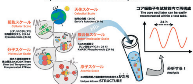
シアノバクテリアの生物時計システム
