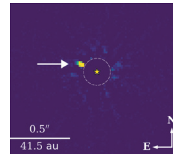
発見された巨大ガス惑星 HIP 54515 b (白矢印)
