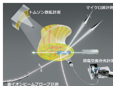
高温プラズマ計測のための代表的な計測装置
