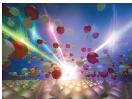
最先端レーザーで観る界面に潜む水分子
