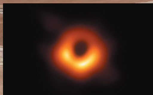
M87銀河中心のブラックホールシャドウ。 国立天文台はこの研究に重要な貢献を果たし、アルマ望遠鏡も観測に参加しました。 (Credit: EHT collaboration)
