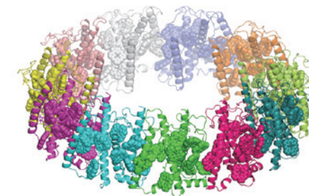
南極の藻類が赤外線で見られるタンパク質の構造
